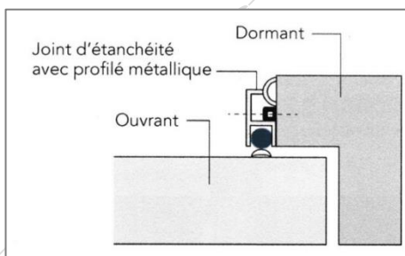
Exemples d'étanchéité à l'air d'ouvrant (Source CSTB)
