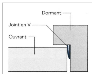
Exemples d'étanchéité à l'air d'ouvrant (Source CSTB)
